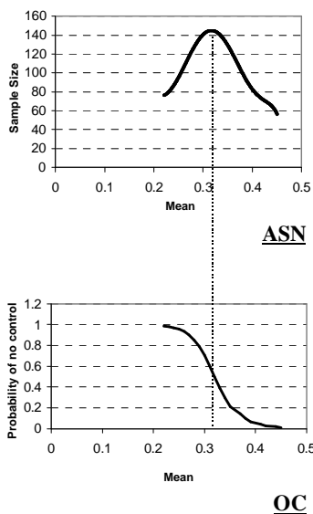
شکل ۴. منحنی‌های ASN و OC سن مادر E. integriceps در طرح نمونه‌گیری دنباله‌ای با استفاده از کادر ۰/۲۵ مترمربع.
