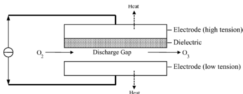
شکل ۱- شکل شماتیکی از ژنراتور تولید ازن به‌وسیله روش تخلیه کورونا.
