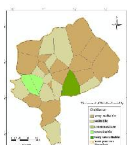
شکل ۶- نقشه‌های حاصل از بررسی مناطق مناسب از نظر رطوبت نسبی Fig. 6. Maps of the study areas suitable for releasing according to the relative humidity
