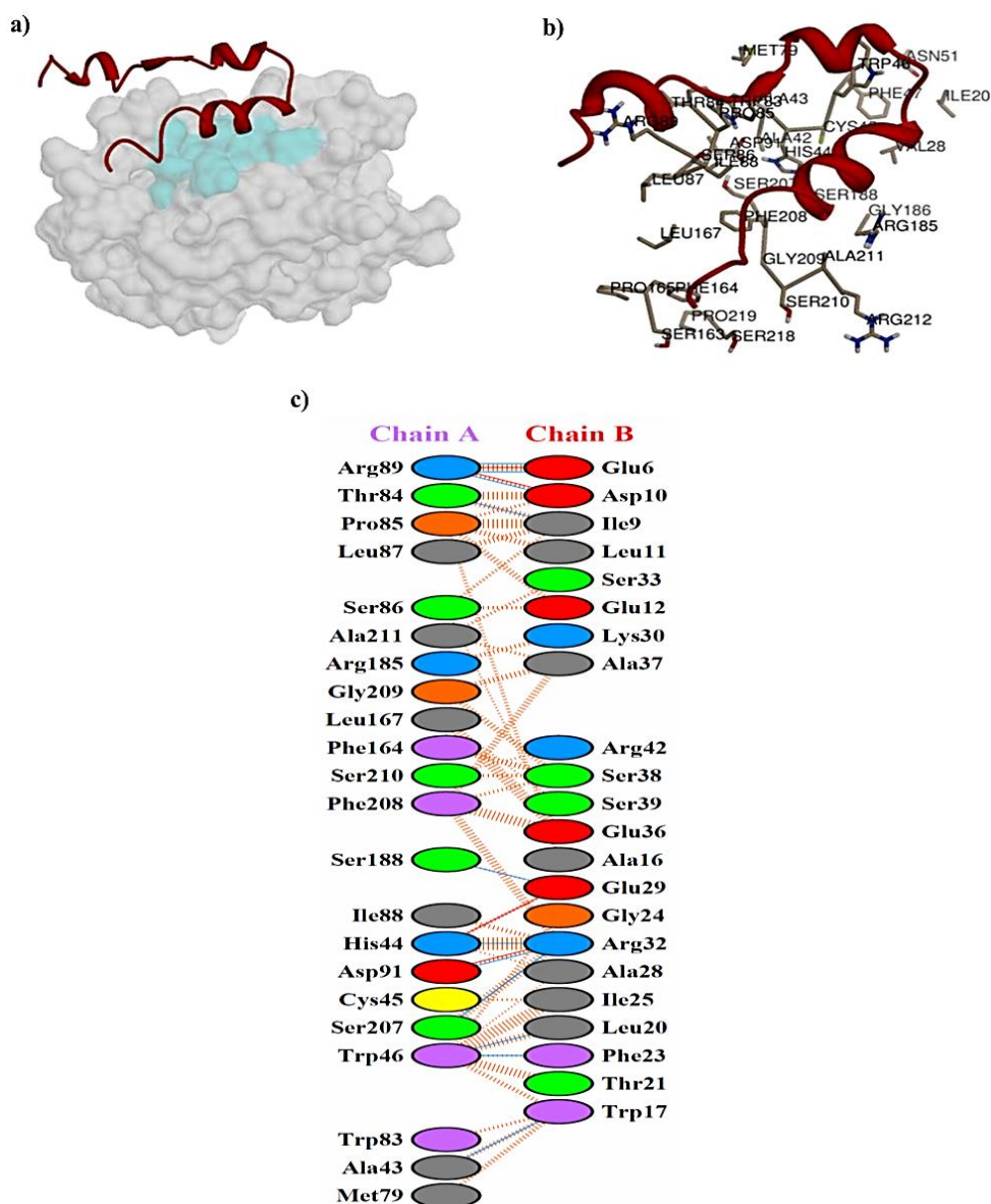
شکل ۴. a ، کمپلکس پروپپتید مهارکننده (قرمز) و آنزیم کیموتریپسین کرم غوزه پنبه (سفید)؛ b ، برهمکنش بین پپتید مهارکننده و اسید آمینه‌های موجود در جایگاه فعال آنزیم و c ، پیوندهای هیدروژنی (خطوط آبی رنگ) و اتصالات غیرپیوندی میان پپتید مهارکننده (زنجیره B) و کیموتریپسین (زنجیره A) معده میانی کرم غوزه پنبه.
