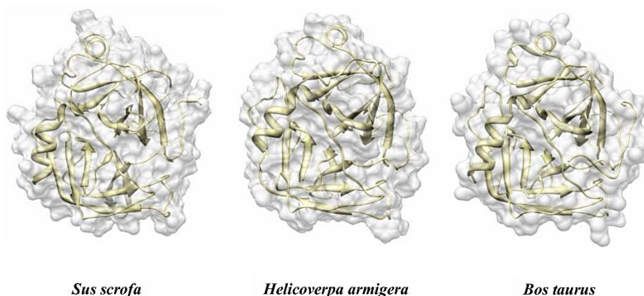
شکل ۳- نمایش فضایی- نواری ساختار سوم کریستاله آنزیم کیموتریپسین Bos taurus و مدل‌های ساختاری کیموتریپسین Helicoverpa armigera و Sus scrofa .
